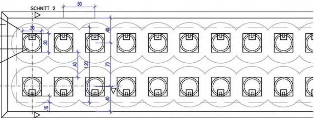
AUFSICHT OHNE PFLANZSUBSTRAT UND EINZEILER 1 M1:20
