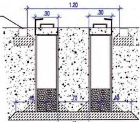
SCHNITT 2 M1:20
