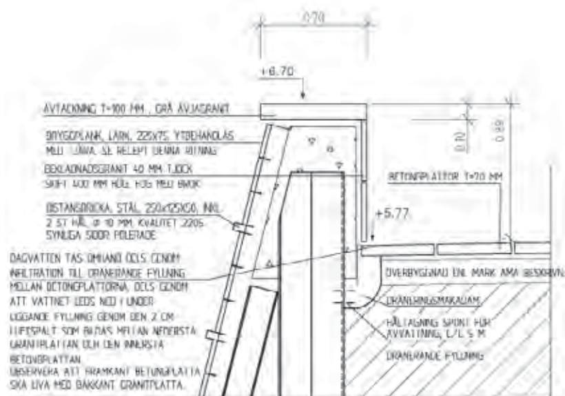
A-A AVBÄARMUR SNITT 120
