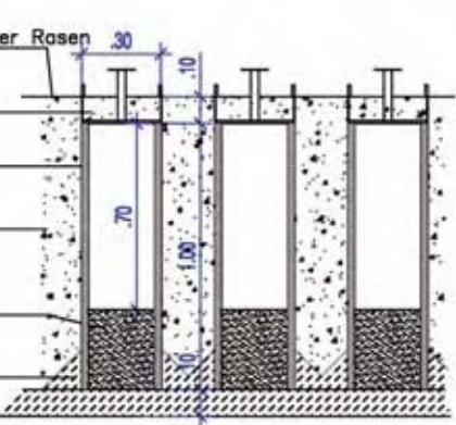
SCHNITT 1 M1:20
